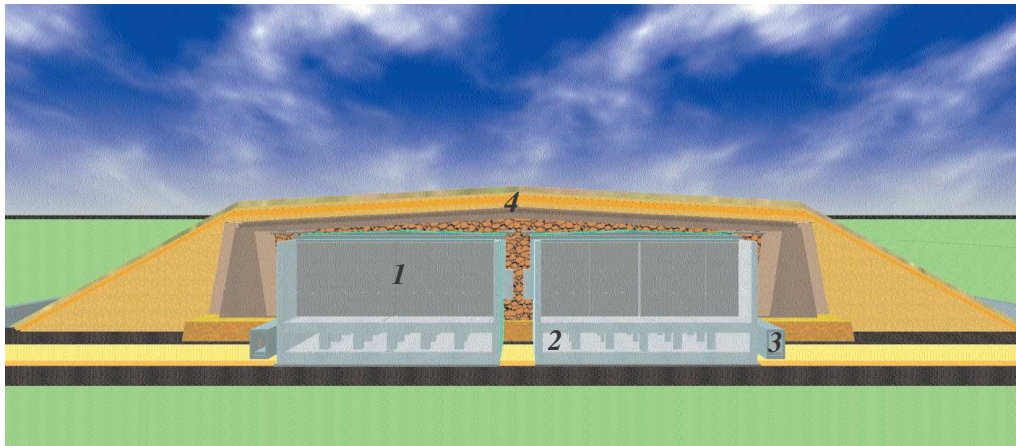
Figuur 2 – Het voorontwerp van oppervlakteberging ontwikkeld door STOLA-Dessel, met één van de twee dubbele rij modules (1), de kelderstructuur (2), de twee inspectiegalerijen (3) en de meerlagige afdeklaag (4) [figuur STOLA-Dessel].
